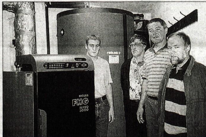
V Turkovi kotlovnici s sodobnim kotlom na polena in s hranilnikom toplote.
