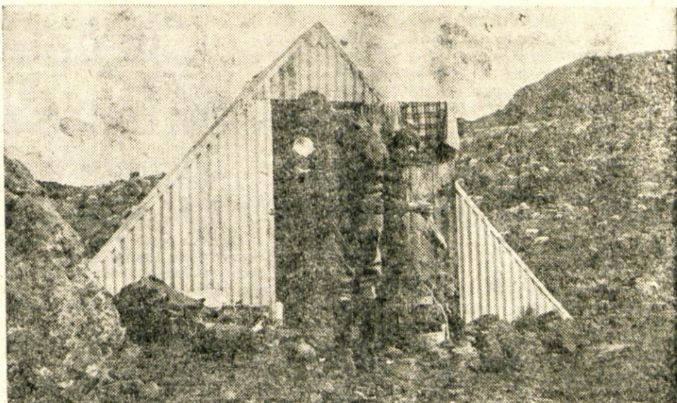
Bivak pod Mawenzijem v višini 4500 m
