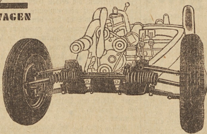
Schwingachse des BMW, Baumuster 326.
