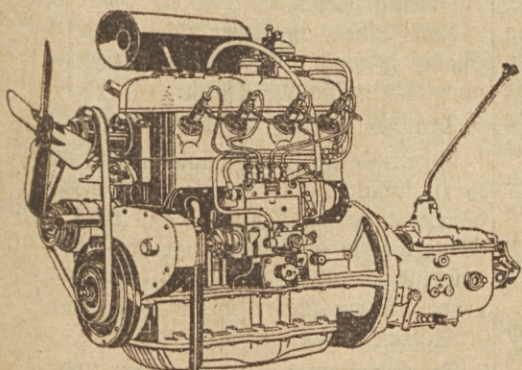
12 Typ 260 D Dieselmotor, Vierzylinder, 2,6 Liter, 45 PS.
