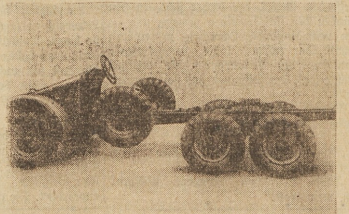
Geländegängiges Krupp-Sechsradfahrgestell Typ L 2 H 243, mit luftgekühltem Krupp Vergasermotor.
