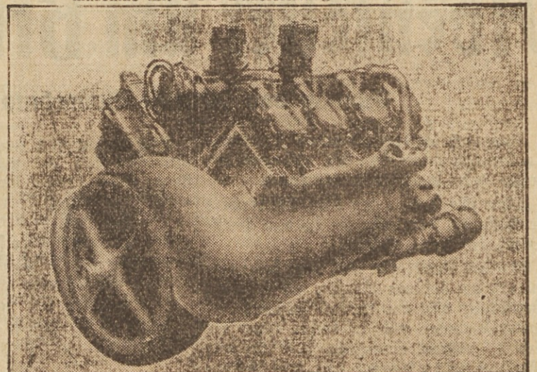
Luftgekühlter 8-Zylinder-Krupp-Vergaser motor, Leistung 125 PS.
