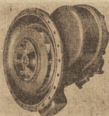
Pumpenrad des Krupp-Strömungsgetriebes A 1, mit verstellbaren Schaufeln. Nach einjährigem Betriebe ist keine Abnutzung festzustellen.
