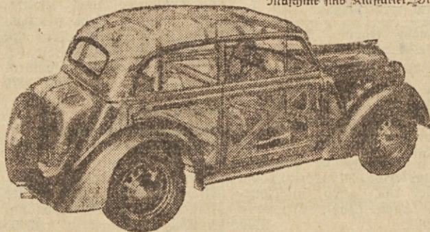
Ein Auto aus Glas! Die gläserne Außenhaut des originellen Modells ermöglicht den Durchblick auf die Stahl-Skelett-Konstruktion, die seit Jahren beim „Olympia“, neuerdings auch beim „Kabett“, von Opel erstmalig in Europa angewendet wird.
