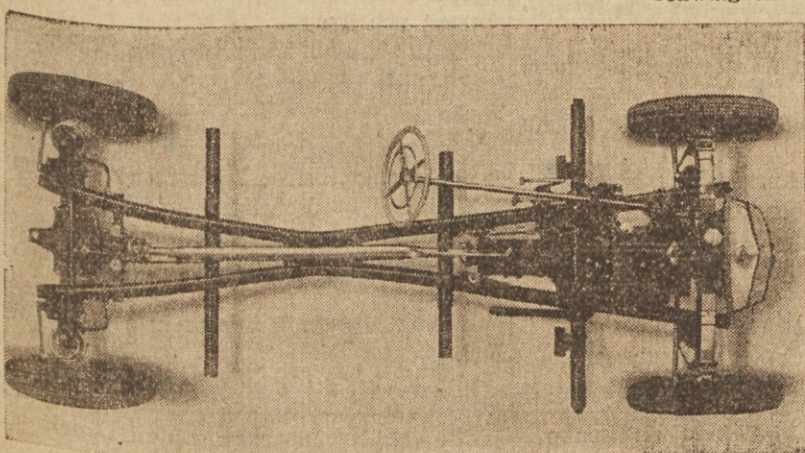
Mercedes-Benz Typ 170 V. Doppelschwingachsfahrgestell.
