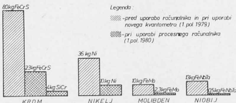
Poprečna poraba ferolegur na šaržo pred uporabo procesnega računalnika in po njej za jeklotvarno ČL 4574 (PK 12 SPL)
