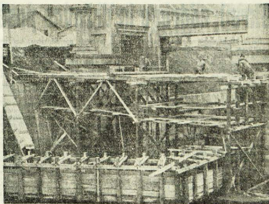
Zamisel, zgraditi zapornico na Ljubljani in s tem regulirati vodo na Barju, je že stara. Leta 1928 so napravili prvi projekt, a do uresničitve ni prišlo, čeprav je bila nadvse potrebna. Zdaj pa je dokončna dograditev vprašanje le 2 ali 3 mesecev. V strugi Ljubljane pri Ambroževem trgu je že pripravljena gradbena jama in prihodnji teden bodo začeli z montažo vodil in pragu. Gladina Ljubljane bo dvignjena ob zapornici za nič manj kot 5 m 89 cm. Sušnih let se barjanec ne bo več treba bati, saj jim bo zapornica avtomatično regulirala talno vodo in preprečevala pogreznje Zapornica bo narejena v tovarni Franc Leskošek in v Litostroju.
