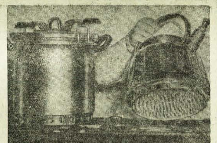
Lonce iz aluminija zaradi svoje praktičnosti že dolgo časa niso nič več novega. Nasprotno pa je nova taka njihova izvedba, da imajo vse dno pokrito s čepki iz iste kovine. Na ta način je ogrjevalna površina trikrat večja, prihranilo plina je 25 do 30 %, čas kuhanja v takem loncu pa je znatno krajši kot v loncu z ravnim dnom. Lonce je napravljen iz enega samega kosa kovine.
