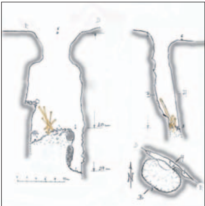
Skica preseka Krimske jame
