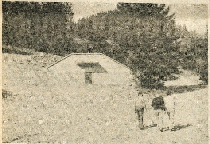
Za zdaj je bilo opravljeno že veliko delo: položen je cevovod od »žrela« do raztežilnika 1 »za vrati« (na sliki) v dolžini 900 metrov in naprej do vodohrana v Zgornjih Gorjušah v dolžini 2360 metrov. Zgrajeni so tudi raztežilniki 1, 2 in 3, od katerih je drugi raztežilnik »na Ravnah« hkrati tudi rezervoar.
