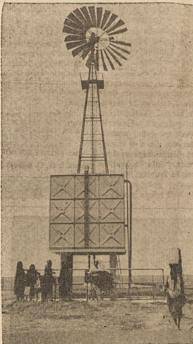
VODA NA VETER — Slika spominja na nekak "mlin na veter", dejansko pridobivajo tu s pomočjo vetra vodo iz globokega studenca. Slika je bila posneta v naselju Gezira v Sudanu.
