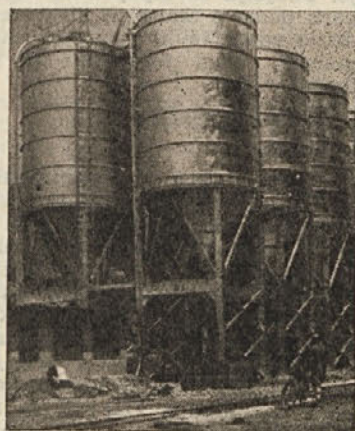
Prekladalna postaja v Gružu s kapaciteto 2400 ton, izdelana v podjetju ITAS
