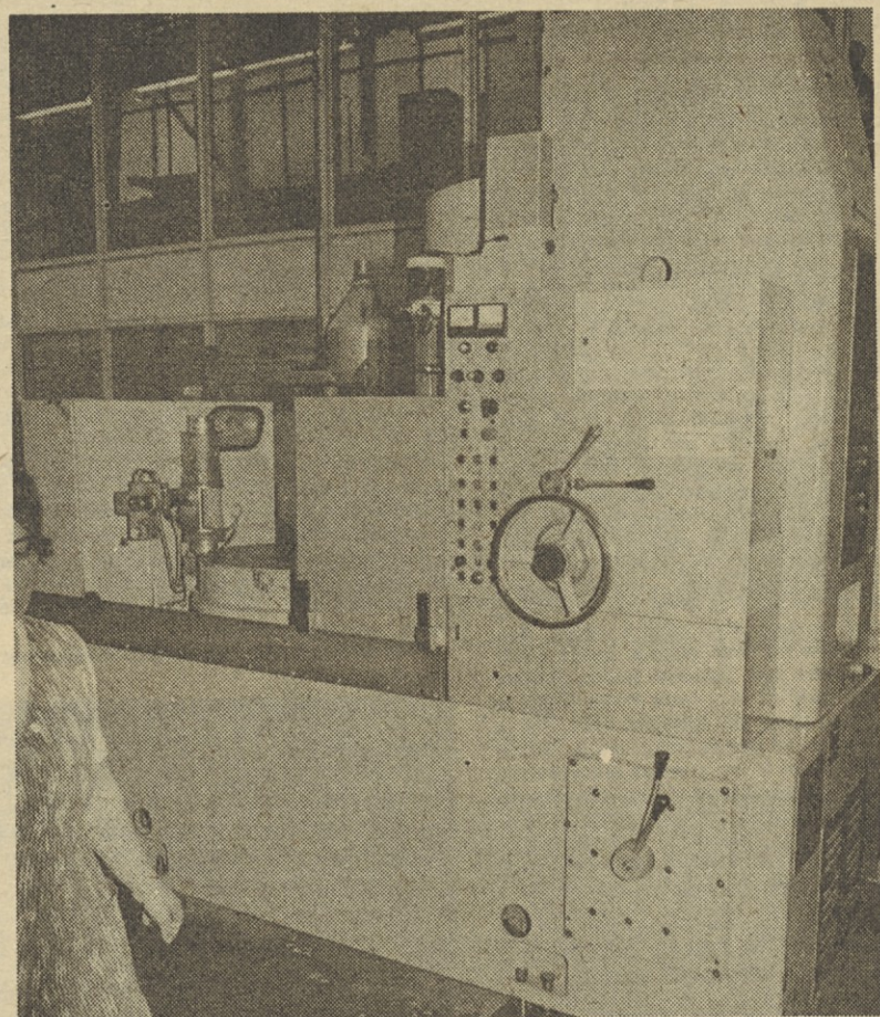
TOZD FERITI: Ta teden so priklopili in začeli uporabljati nov ploškovni brusilni stroj uvožen iz SZ. Služil bo za brušenje feritnih izdelkov. Tako so bistveno povečali kapaciteto v tej fazi obdelave in dosegli večjo zanesljivost in kvaliteto.
