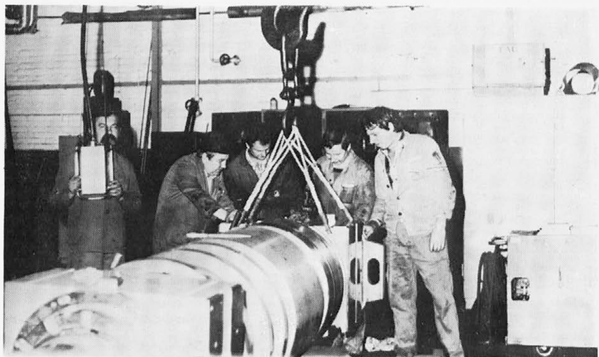
Ko so valji na mizi, ne na progi — obdelava in montaža bistvenih delov težke proge v delavnici valjev v Valjarni
