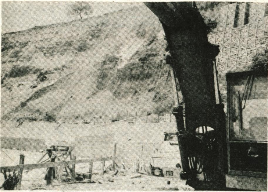
Glavna dela na izkopu 14 metrov širokega in 12 metrov globokega vodnjaka 45 metrov pod jezo elektrarne so se začele sredi junija. 25. avgust je rok, ko mora 25-članska Gradbinčeva gradbena ekipa končati z deli, potem pa bo Metalna začela z montažo jeklenih oblog in vodil za vgradnjo pomožne zapornice.
