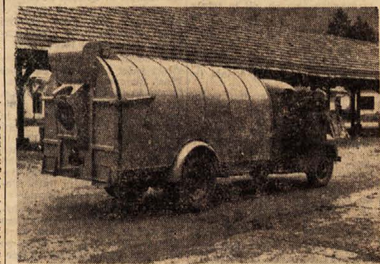
Eden izmed avtomobilov, s kakršnimi bo »Snaga« odvažala prihodnje leto iz središča Ljubljane smeti. Izdelal ga je SKIP iz Vizmarij
