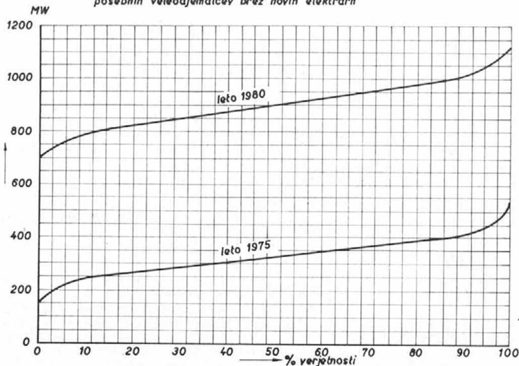
Primanjkljaji moči v Sloveniji v času konice pri polnem obratovanju posebnih veleodjemalcev brez novih elektrarn
