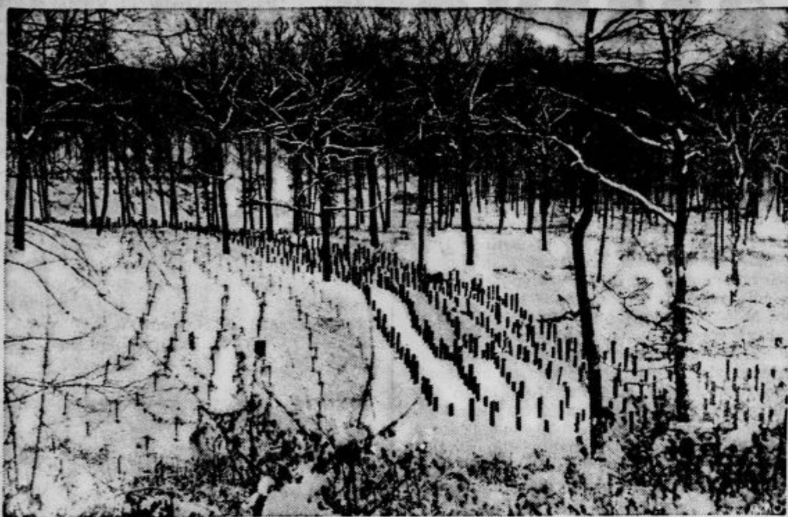
Protitankovske ovire na francoski strani
