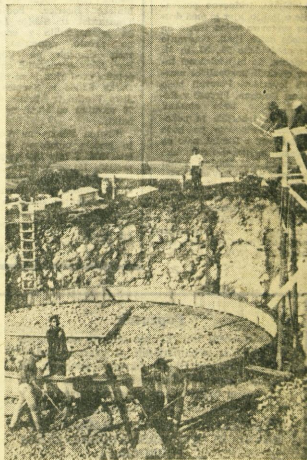
REZERVOAR NA KAMNITNIKU — Dela za ureditev škofjeloškega »vodovodnega problema« so v teku. Najprej bodo uredili rezervoar na Kamnitniku, v katerega bodo preko noči črpali vodo, da bo tako lahko čez dan oskrboval višje ležeče kraje ter tako razbremenil vodovodno omrežje v konicah. Foto — F. Perdan
