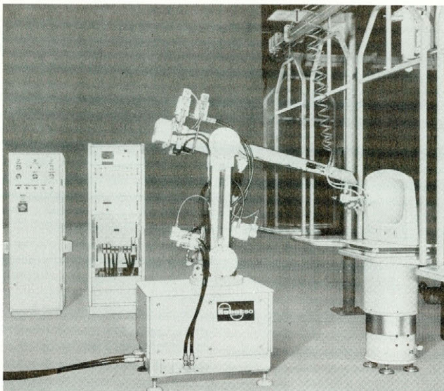
Robot 50 — pri glaziranju sanitarne Keramike v poskusnem obratovanju
