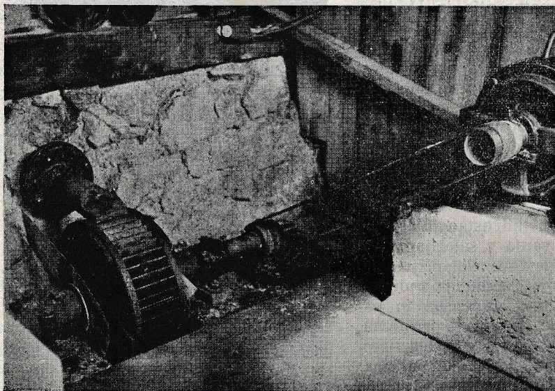
Turbina in dinamo naše „centrale“.
