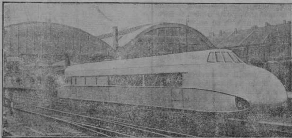
Prva vožnja »Zeppelina« na tračnicah. — Voz na pogon s propelerjem je na tračnicah prestal dne 10. majnika poskušnjo vožnjo in dosegel brzino 205 km na uro.
