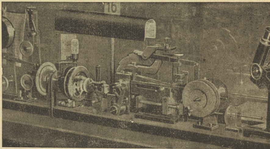
Na teh silno kompliciranih strojih izdelujejo zavojke. Paznik pa nadzoruje skozi mikroskop na desni.
