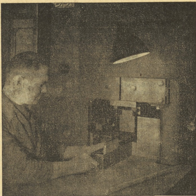
Hidravlične stiskalnice, ki izdelujejo iz volframevega praha kovinske palice.
