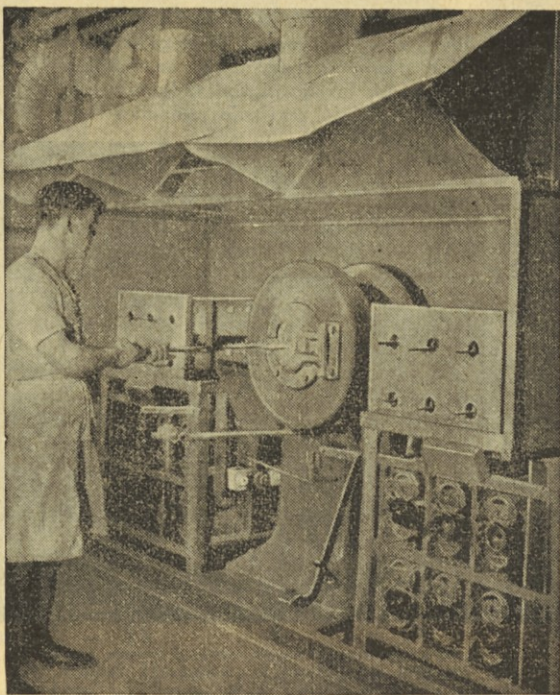
To so strojna kladiva, ki udarja o 6000 krat v minuti in izpreminjajo palice v 1 mm debelo žico.
