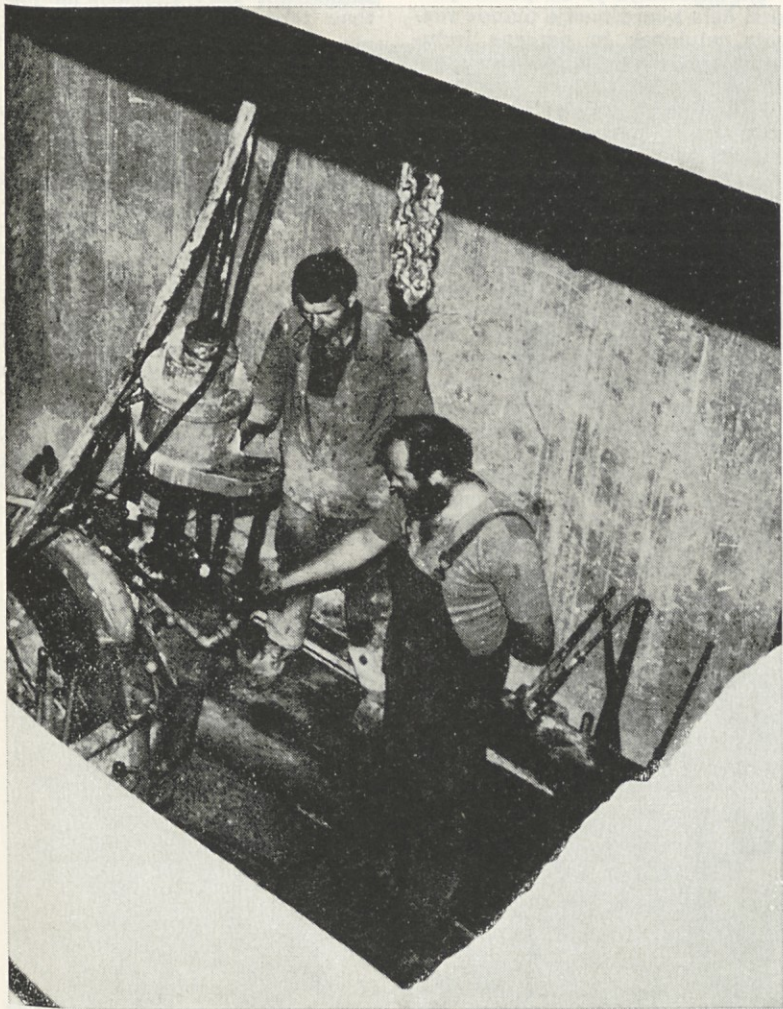
Gradbena dela ureditve osnovnega ležišča za generator in turbino so bila zelo zahtevna in odmerjen jim je bil silno majhen manevrski prostor v devet metrov globoki »luknji«
