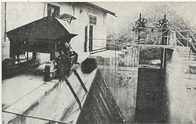
Star čistilni stroj HE Fužine je svoje že odslužil; zamenjal ga bo nov, ki bo imel večjo čistilno kapaciteto in bo omogočal boljši izkristek vodne mase
