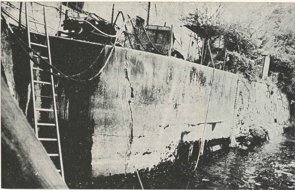
Zob časa in vpliv vode sta na stoletnem obrežnem fužinskem zidu pustila svoje sledove; potrebna je bila sanacija
