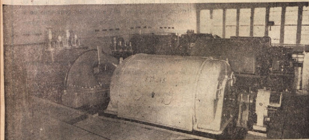
Strojnica za turbogeneratorje v elektrarni Trbovlje
