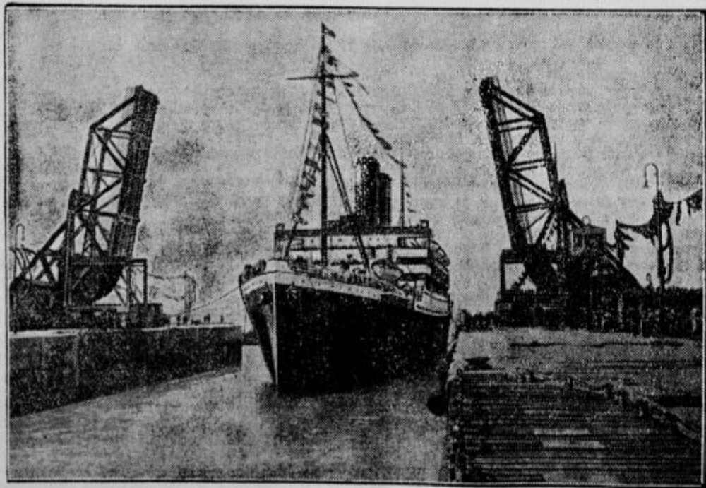
Otvoritev največjega angleškega doka v londonskem pristanišču, ki je stal 560 milijonov dinarjev. Dolg je 304 m. širok 33,5 m in globok 13,7 m. Izpraznitev odn. polnitev doka traja komaj četrt ure.
