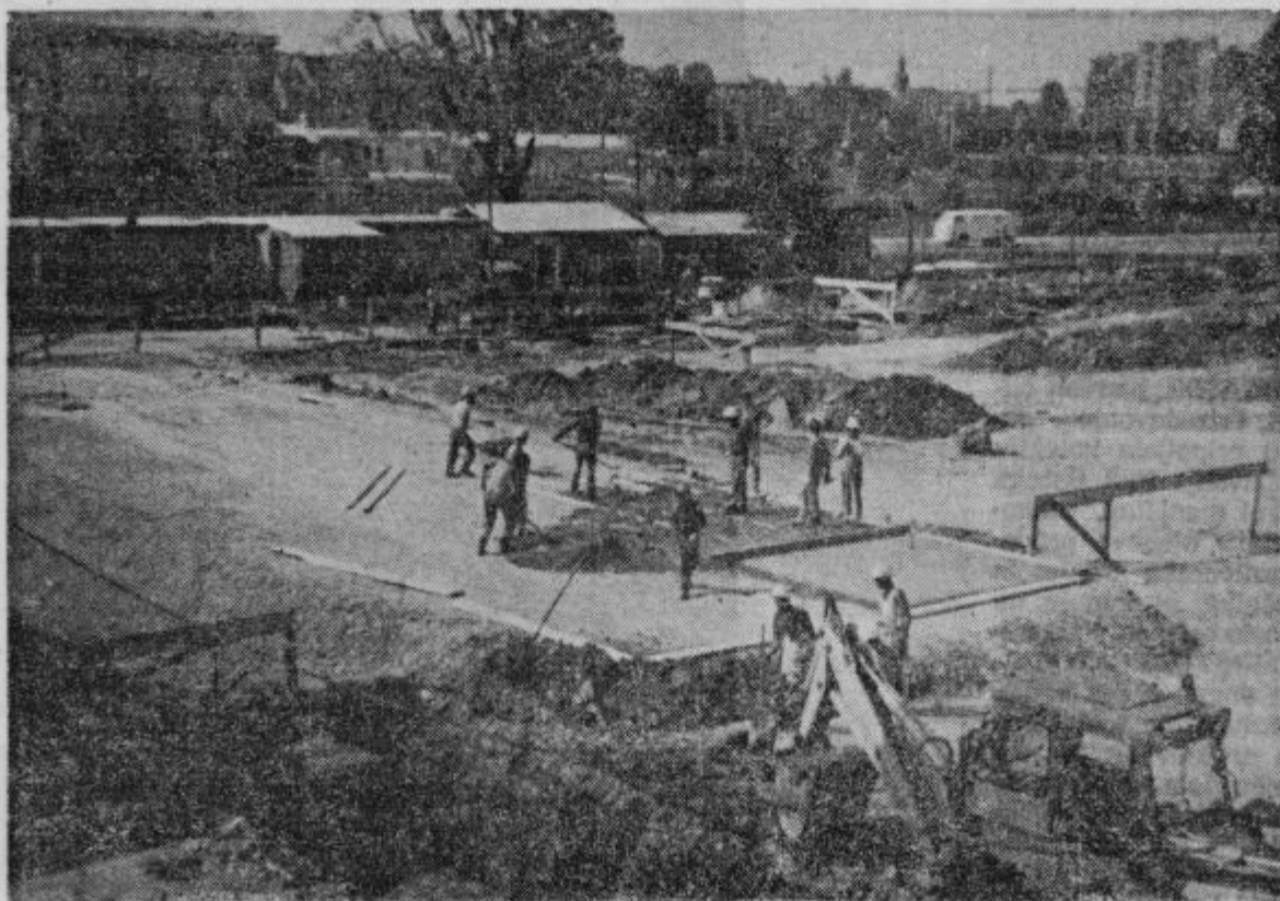
Gradnja nove proizvodne hale, ki bo omogočila boljše delovne pogoje, boljše delovne rezultate in kvalitetnejši razvoj.
