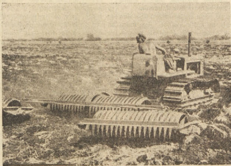
Potem, ko je zemlja preorana in posejana, pride na vrsto strojna brana, ki ima veliko zmogljivost in opravi delo hitro in vestno.
