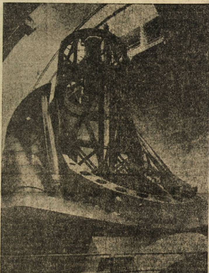
HALEJEV DALJNOGLED — Največji daljnogled sveta je Halejev reflektor v zvezdnari na gori Palomar v Kaliforniji, ki ga predstavlja slika. Daljnogled ima 508 cm v premeru, tehta 530 ton in sloni na tako gladkih krogličnih ležajih, da ga lahko premika mali elektromotor z eno dvajsetinko konjske sile, ko zasledujejo skozi njega zvezde premičnice v razdalji do ene milijarde svetlobnih let. Zrcalo na dnu njegove cevi, ki tehta 14 in tričetrt tone, so brusili 8 let. Halejev teleskop je last kalifornijskega tehnološkega zavoda.
