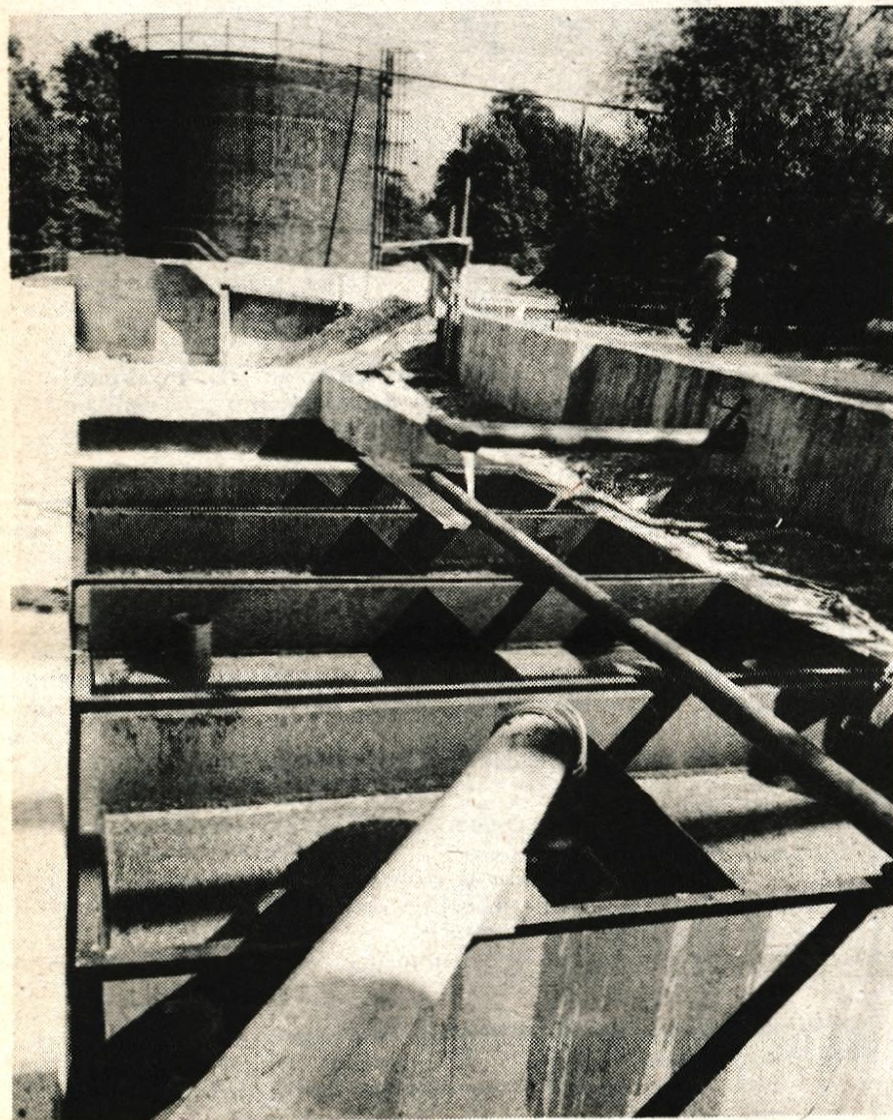
Sistem prekatnih bazenov, ki jih Oljarica zdaj uporablja, da lovi odpadke proizvodnje, bo z novo tovarno margarine moral zamenjati sodobnejši in tehnološko primernejši način varovanja okolja. — Foto: F. Perdan
