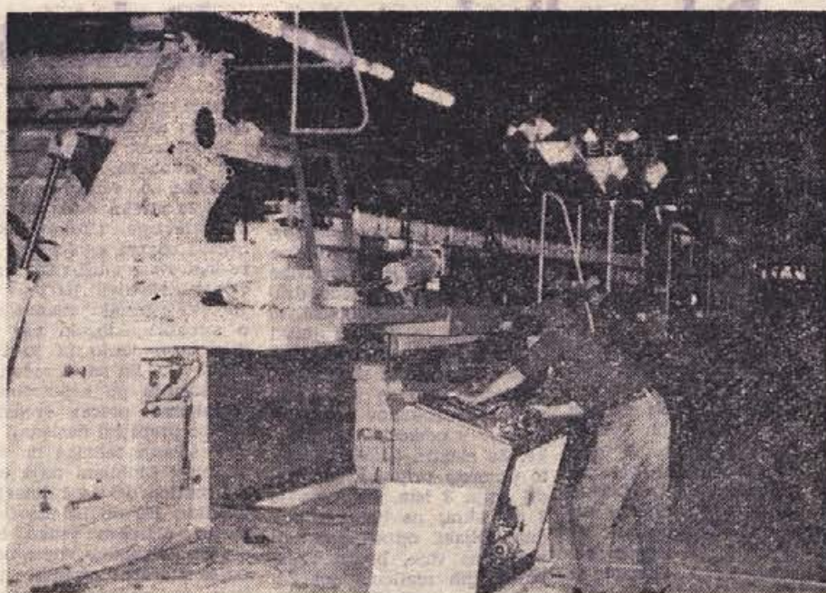
Pogled na majhen del novega papirnega stroja — velikana v zadnjih dneh montaže in preizkušanja
