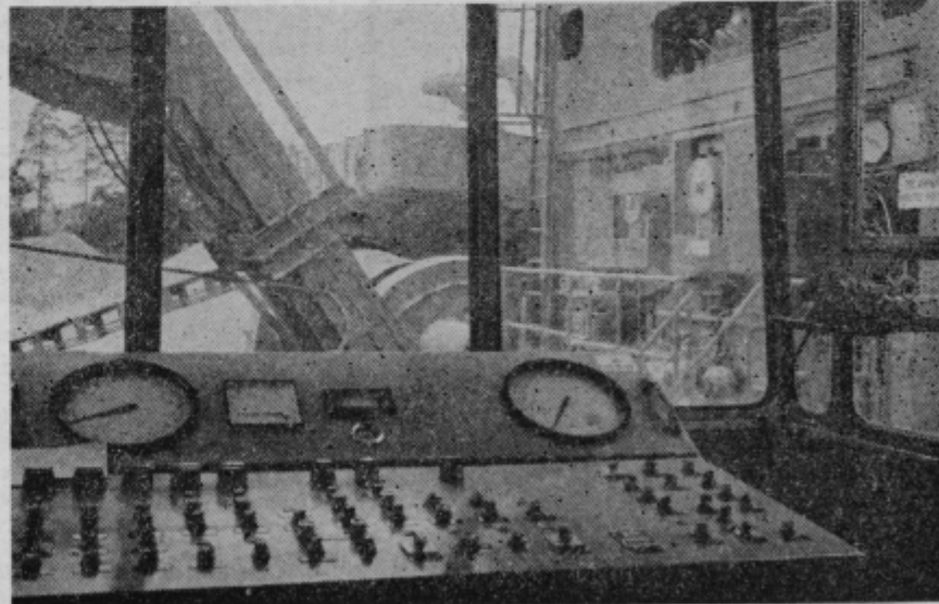
Libelina procesna tehtnica v asfaltni bazi Pirešica (skozi okno se vidi dvigalo)
