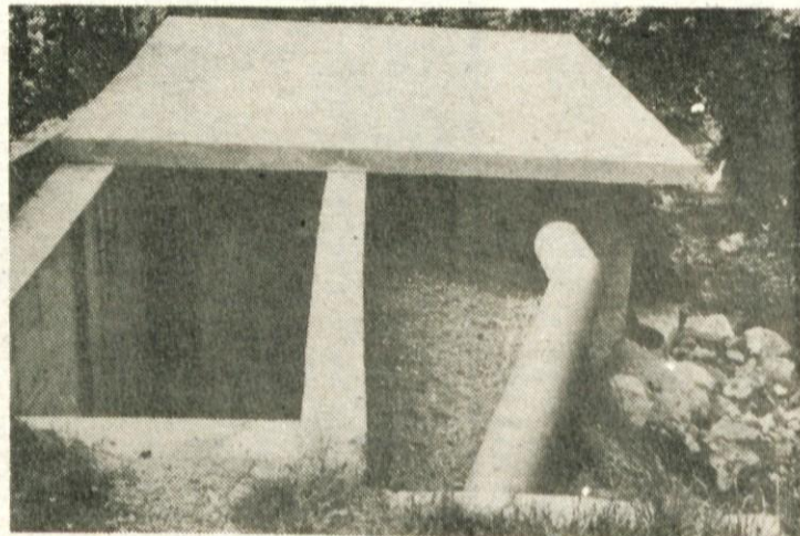
Elektrikarji Elektro Gorenjske so bili presenečeni nad brezhibno opremo in gradnjo majhne hidrocentrale v Ratečah. — Foto: F. Perdan
