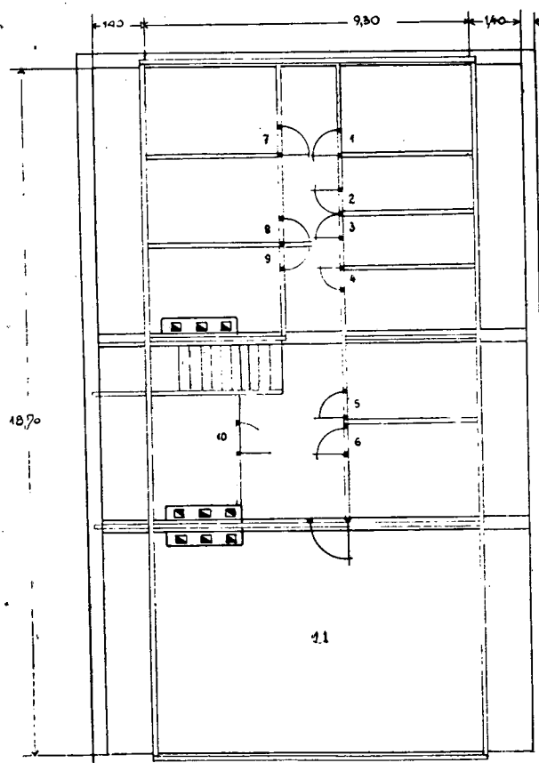
Sl. 6. Loden (h. št. 6). — Veža v prečni osi stavbe z mestjami (1—6) in dohodom z brega (7). Prim. sl. 4
