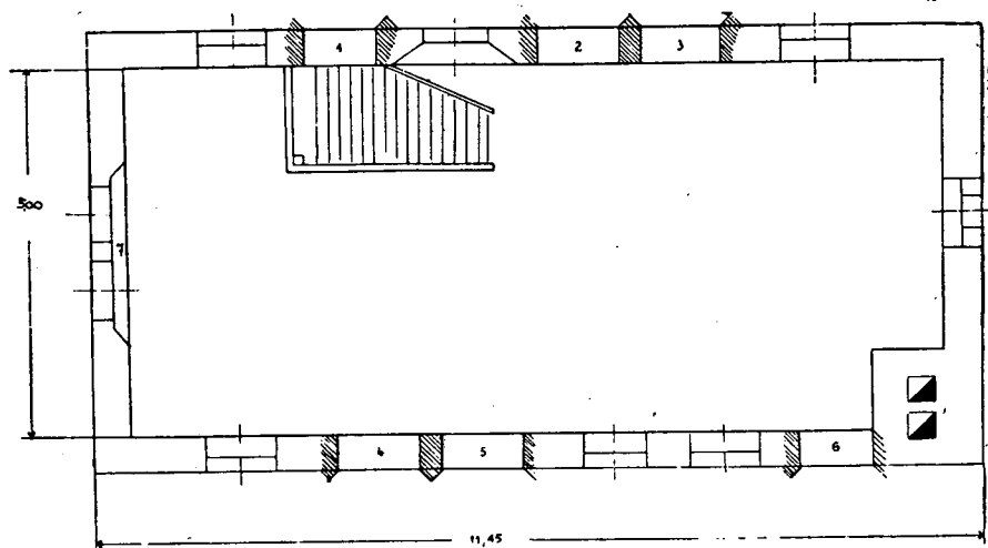
Sl. 6. Loden (h. št. 6). — Veža v prečni osi stavbe z mestjami (1—6) in dohodom z brega (7). Prim. sl. 4
