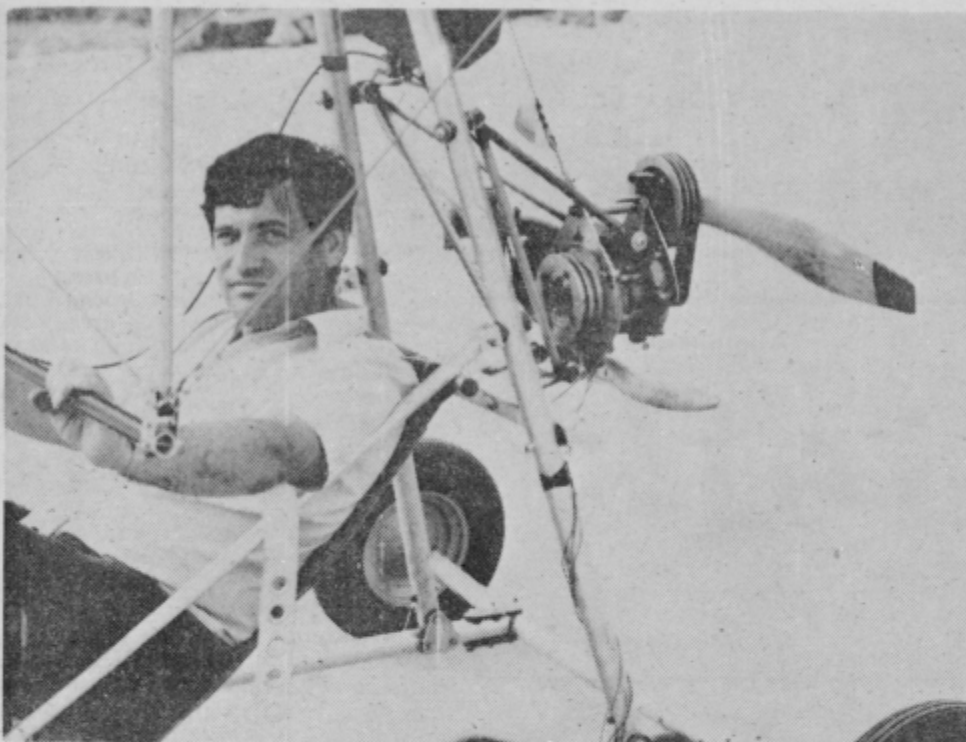
Janko Žličar na »pilotskem« sedežu. Spodnji del oziroma podvozje zmaja je narejeno iz lahkih kovin, cevi pa so na najbolj obremenjenih mestih ojačane. Zada je motor »Prima«, na fotografiji pa je še star, dvokraki propeler. Novi, trikraki, se je bolj obnesel in izkoristek je precej večji.
