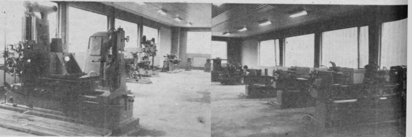
Pogled na novo proizvodno dvorano. Na levi v ospredju horizontalno vertikalni stroj, edini te vrste v ptujski občini. V ozadju na desni strani stroja za ozobljanje stožčastih in poševnih zobnikov — specialnost Gomilškove delavnice.
