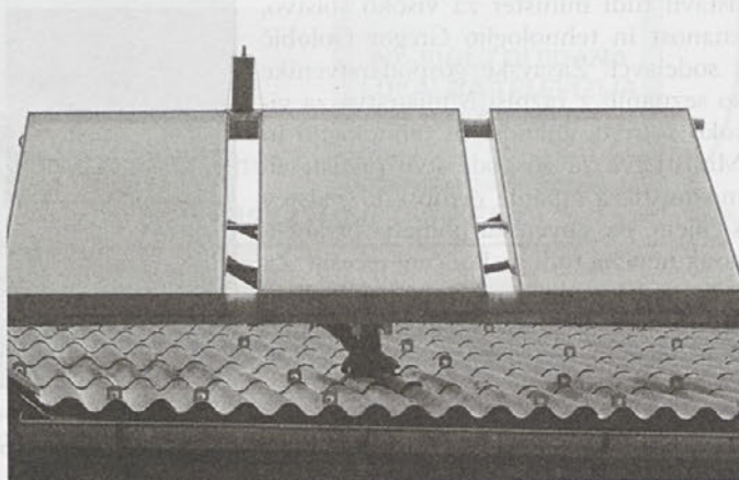
Sončni kolektorji s sledilno napravo (sledijo gibanju sonca), ki jo je izdelal lastnik sam.
