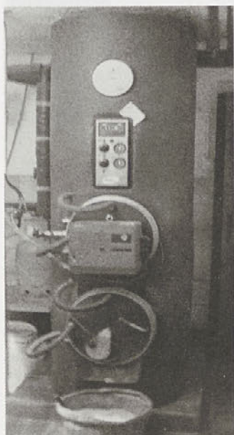
Peč, kjer se lahko uporablja več energentov: drva, kurilno olje, toploto iz sončnih kolektorjev.
