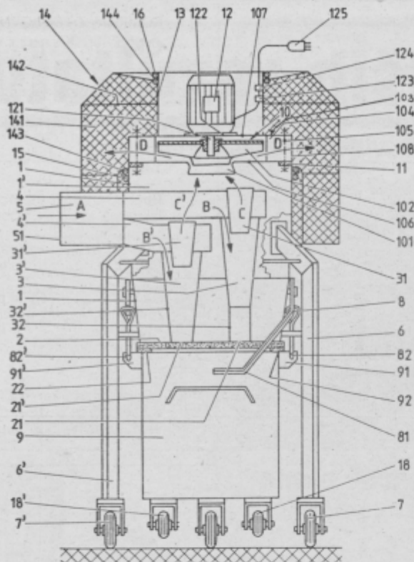
Multiciklonski izločevalnik s filtrom - MCF-1800/2.2.
