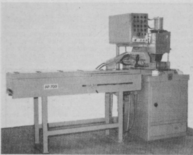
Avtomatska žaga za hladen razrez.
