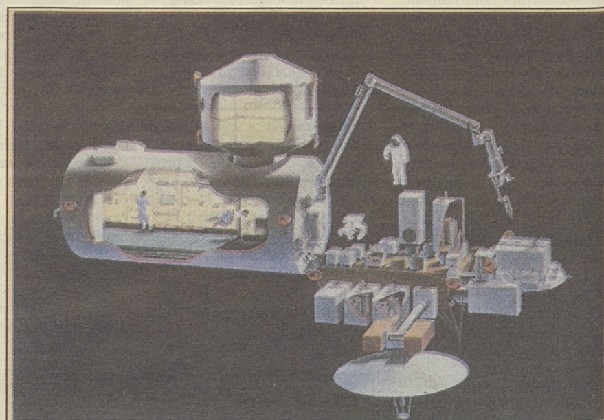
Pogled na japonski Eksperimentalni Modul - JEM sesavljen iz treh glavnih delov. Laboratorijskega modula, v katerem bodo vesoljci - znanstveniki izvajali poskuse in upravljali mehansko roko pri delu na eksperimentalni platformi, ki predstavlja drugi del JEM-a. Tretji del je eksperimentalno logistični modul, pritrjen nad laboratorijski modul, ki bo služil kot skladišče za raznovrstne vzorce. Preko njega po potekal njihov transport na relaciji Zemlja - JEM - Zemlja.
