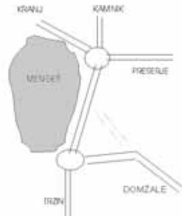
Predlog obvoznice s samo dvema krožiščema
