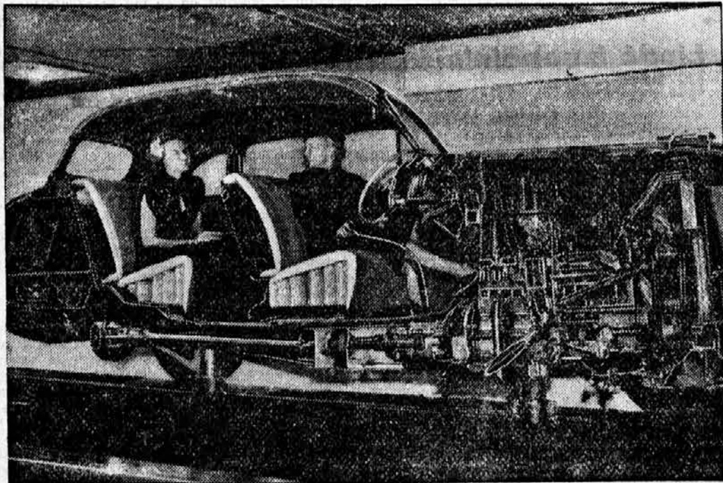
Prerez avtomobila, ki je razstavljen v New Yorku.
