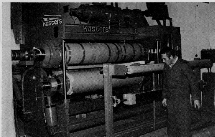
Kalander firme Küsters za dosego različnih efektov na tkaninah
