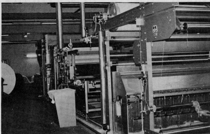
Sanforizirni stroj na katerem dosegamo mehansko skrčenje tkanin. S tem postopkom se prepreči nadaljnje krčenje tkanin pri gotovih izdelkih
