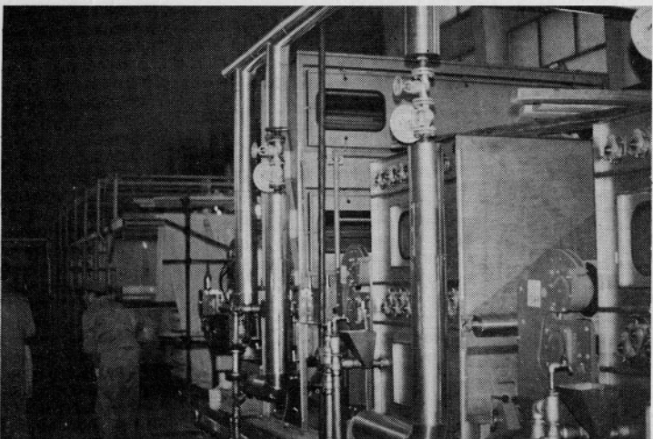
Spremenjen način beljenja in možnost izpiranja tkanin po razškrbljenju in ostalih obdelavah bo močno pocenil in izboljšal proces obdelave tkanin
