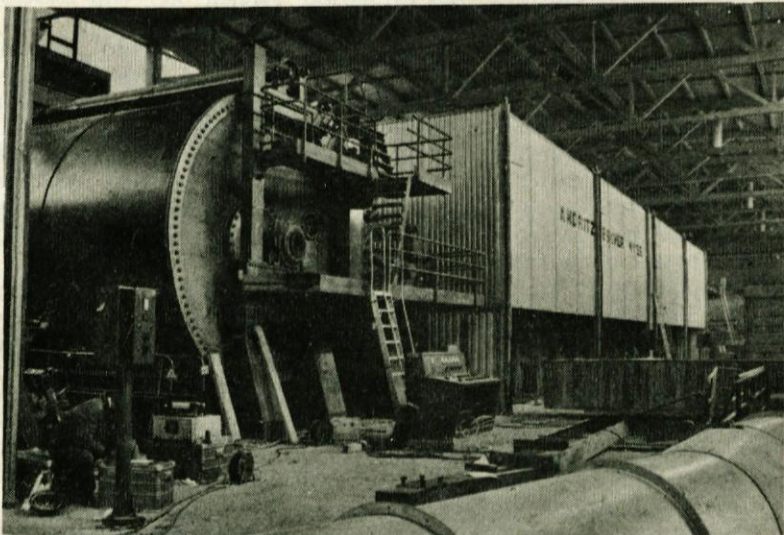
V Papirnici Količevo potekajo montažna dela opreme za kartonski stroj III. Na sliki vidimo gladilni valj, ki je med najtežjimi deli nove opreme
