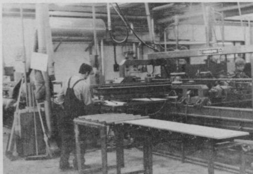
Malone vsa dela opravljajo specialni mizarški stroji, ki so med seboj povezani s tekočim trakom, ki prenašajo izdelke od faze do faze v strojni obdelavi.
