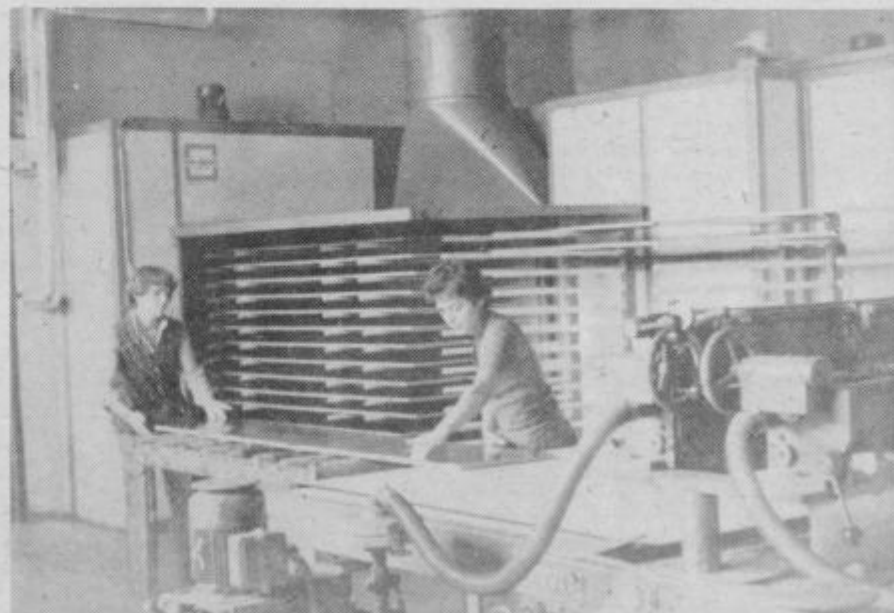
V lakirnici je komajda zaznavan vonj po lakih, saj jih odzračevalne naprave povsem izsesajo iz prostora. Ročno prenašanje takšnih plošč na sušilne police je najtežje breme, ki ga je treba dvigovati.
