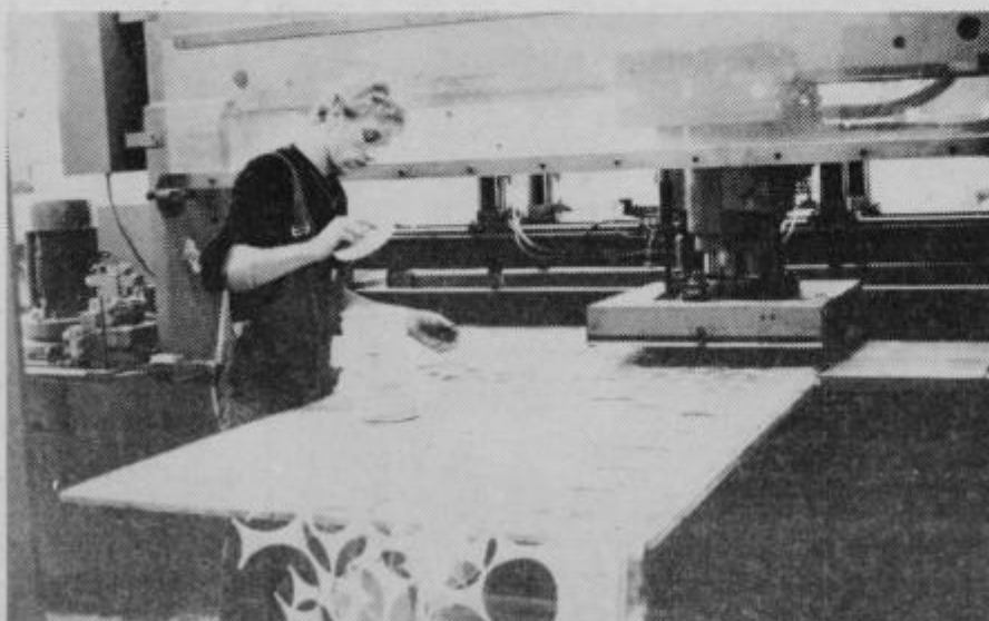
Izsekovalni stroj vodi računalnik, ki omogoča za 10 odstotkov večji izkoristek.
