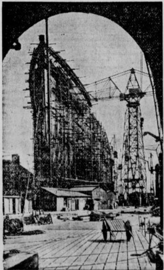
Znano angleško brodersko podjetje Cunard-White-Star-Line gradi največjo ladjo na svetu, ki bo obsegala 75.000 ton. Gradnjo so lansko leto prekinili radi pomanjkanja denarja, zdaj nadaljujejo z delom. Anglija upa, da si bo s to ladjo zopet osvojila modri trak, to je odklovanje za najhitrejšo vožnjo med Evrazo in Ameriko.
