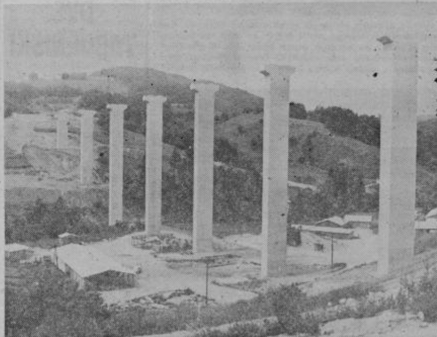
Viadukt Pletovarje
