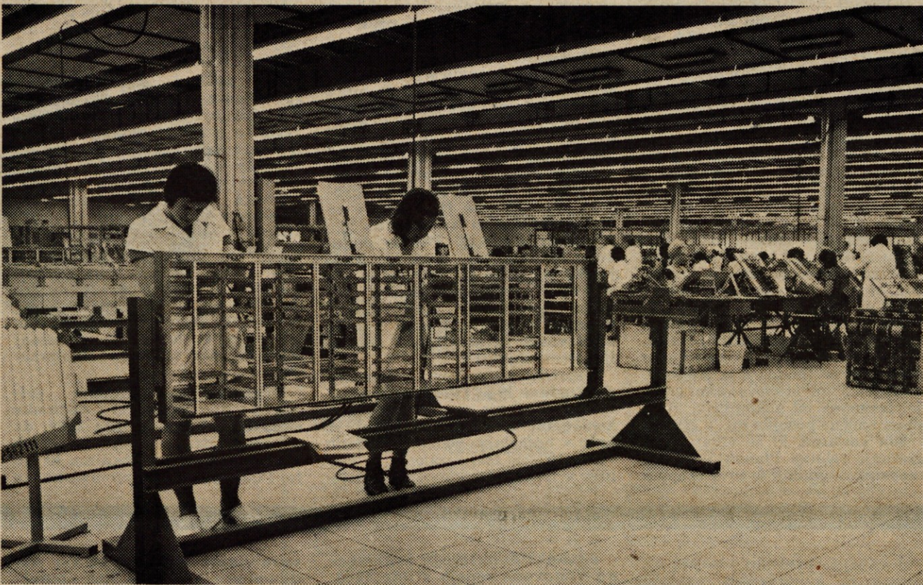
Spajanje novih stojal elektronske centrale Iskra 10 C
