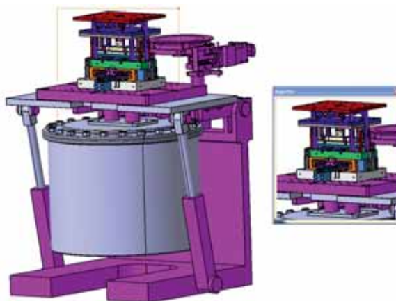
Koncept nizkotlačnega litja z dvema livnima cevema
