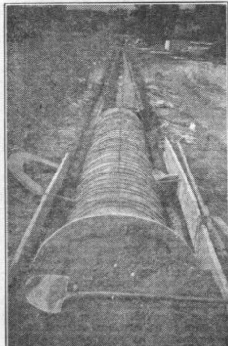
Betoniranje velikega kanala pri kanalizaciji Rožne doline.
