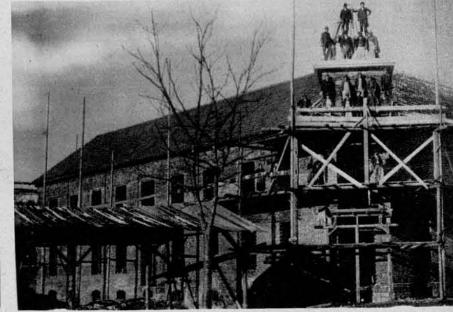
Društveni dom v Šoštanju, ki bo eden največjih v Sloveniji. Graditi so ga začeli 11. IX. 1925 ter je bil ob Novem letu že pod streho (stavbenik g. D. Korošec).
