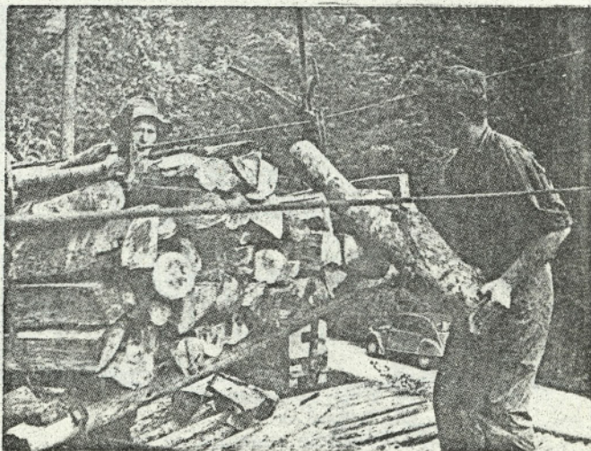
Gravitacijska žičnica je pripeljala tovor drv - foto GG Bled.
