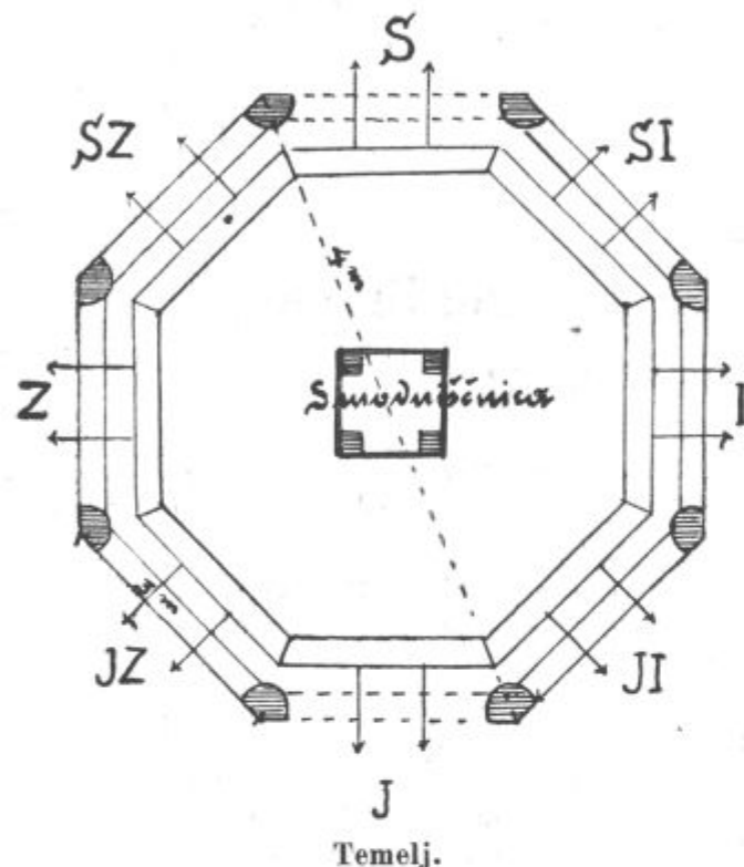
II. črtež za streljarno (bajto).
