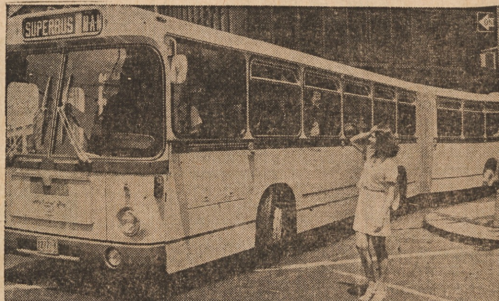
NOVA VRSTA AVTOBUSA — Slika kaže "superbus" na cesti New York Cityja, izdelan v Zahodni Nemčiji. Bus je nekaj ožji od ameriških, pa 14 čevljev daljši. Za lažje zavijanje ima v sredi gumijasti vložek, ki omogoča krivitev vozila na ostrih ovinkih. Avtobus stane $85,000 in ga preskušajo. V njem je prostora za 63 potnikov.
